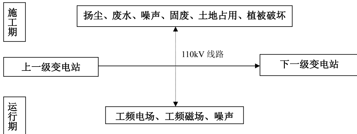
图 1、110kV 输电线路工程工艺流程及产污环节示意图
